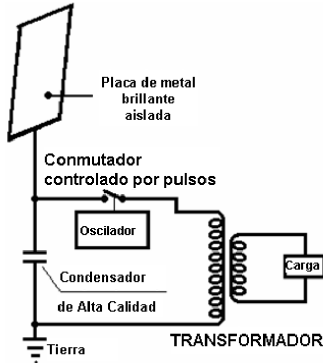
Sistema de Antena con Placa Brillante Aislada de Nicola Tesla
