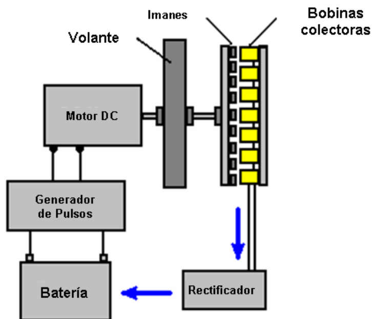
Diagrama del dispositivo de John Bedini
