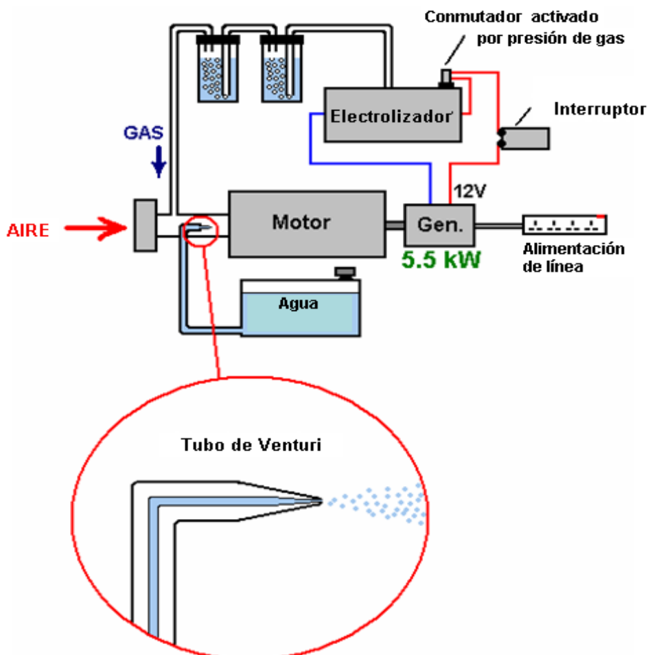
Diagrama del sistema usado para modificar el Moto Generador
