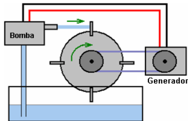
Diagrama del sistema de rueda de paletas
